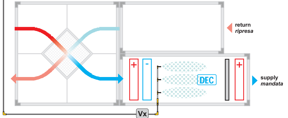
V = SOLENOID VALVES DRAIN KIT - ELETTROVALVOLE SCARICO
